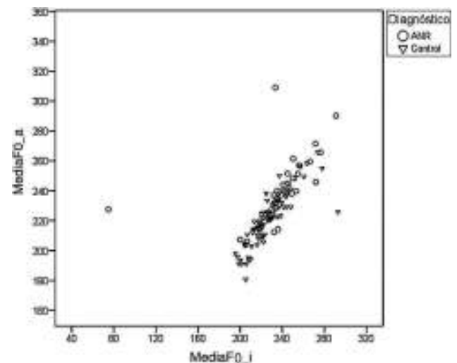
Figura 1. Diagrama de dispersión entre la frecuencia fundamental para la "a" y para la "i".
