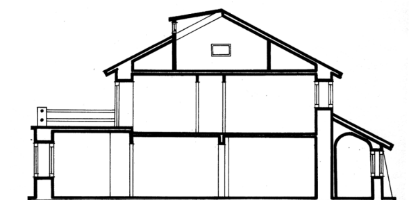
Fig. 9 - Sección Escala 1:100
