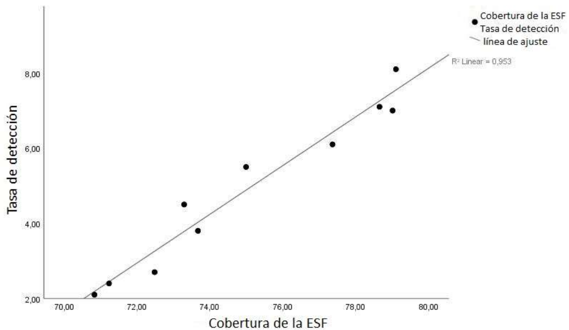
Figura 2: Diagrama de dispersión simple que muestra la correlación entre la cobertura de la ESF (%) y la tasa de sífilis congénita por mil nacidos vivos con una línea de ajuste, Nordeste, Brasil, 2008-2017.
