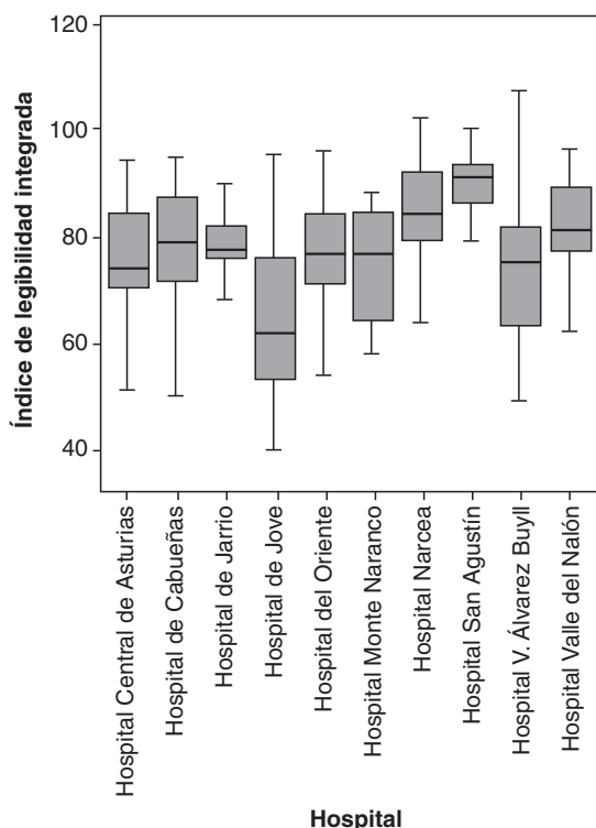
Figura 1. Variabilidad para la legibilidad de los consentimientos informados entre los hospitales de Asturias.
