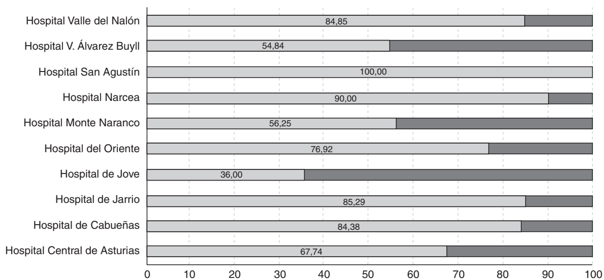
Figura 2. Porcentaje de DCI con una legibilidad aceptable (ICO ≤ 30 y LEGIN ≥ 70).
