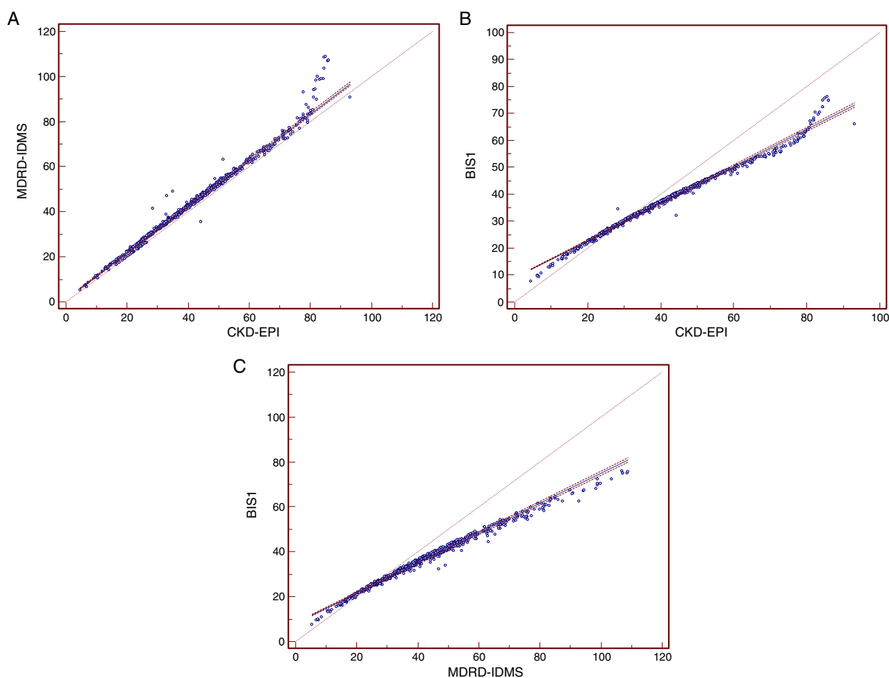
Figura 2 – Rectas de regresión de Passing Bablock de las ecuaciones de filtrado glomerular. Rectas de regresión de Passing-Bablok entre las distintas ecuaciones para la estimación del filtrado glomerular. A) Recta de regresión MDRD4-IDMS -CKDEPI. B) Recta de regresión BIS1-CKDEPI. C) Recta de regresión.
